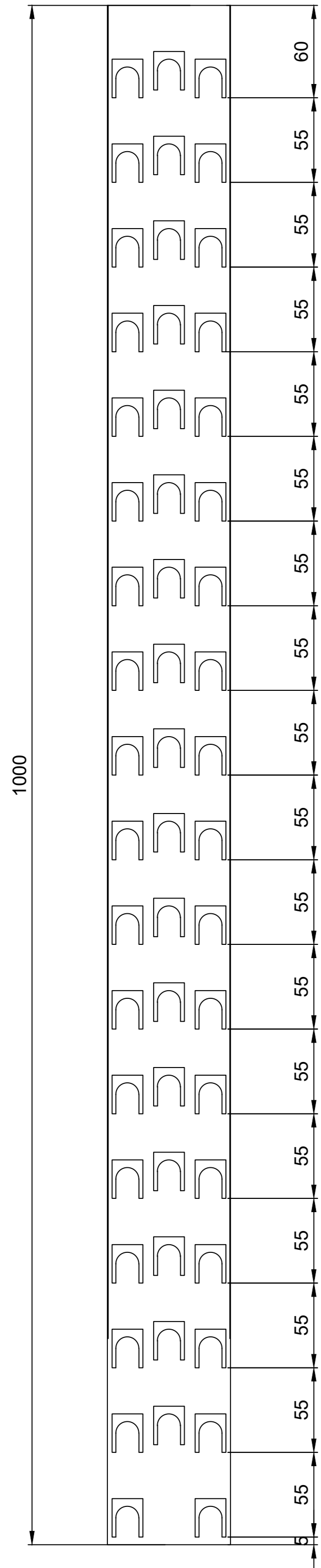
18 Lamellen
