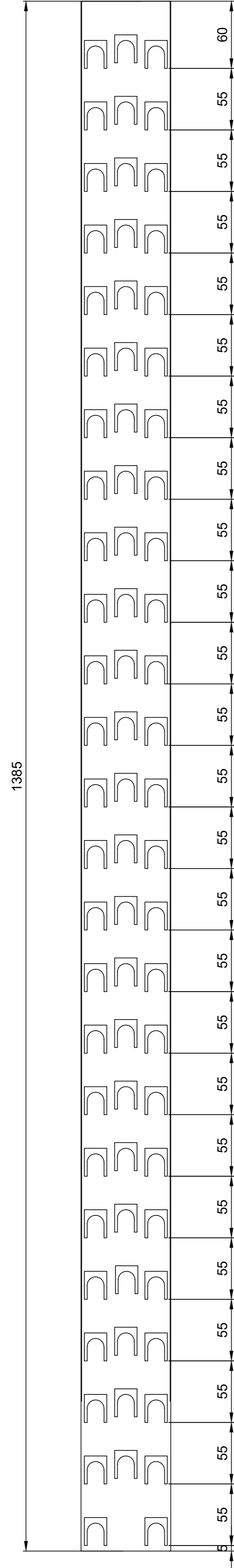
25 Lamellen
